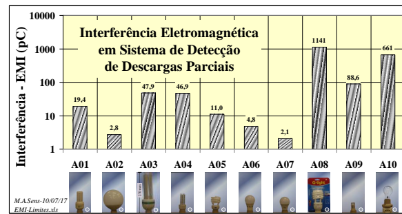
Figura 5 - Perturbação Eletromagnética
